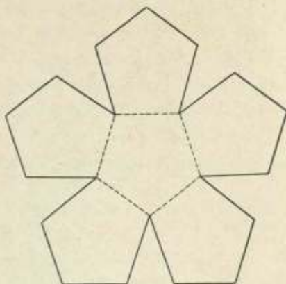
DODECAHEDRON.
