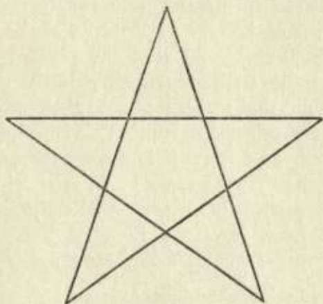
FIG. 9. The Pentagram.
