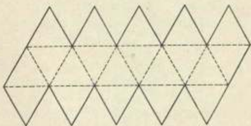
ICOSAHEDRON.
