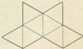
OCTAHEDRON.
